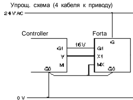
Аналоговое упр., 16 V DC питание для контроллеров (TAC 218E/RM, TAC 221L, TAC 228R/RL/RF, TAC 239W, TAC 258R/RL, TAC 268R/RL/RF)
