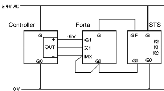
Станд. схема (5 кабелей к приводу)
