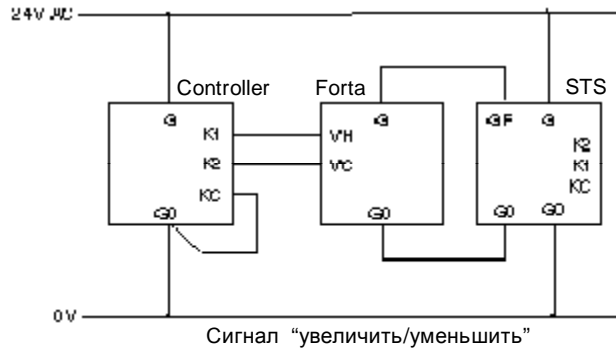
Станд. схема (4 кабеля к приводу)
