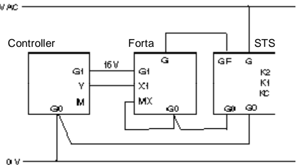
Аналоговое упр., 16 V DC питание для контроллеров (TAC 218E/RM, TAC 221L, TAC 228R/RL/RF, TAC 239W, TAC 258R/RL, TAC 268R/RL/RF)
