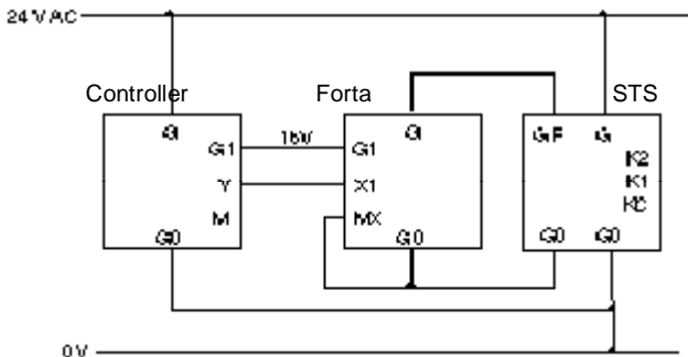
Аналоговое упр., 16 V DC питание для контроллеров (TAC 218E/RM, TAC 221L, TAC 228R/RL/RF, TAC 239W, TAC 258R/RL, TAC 268R/RL/RF)
