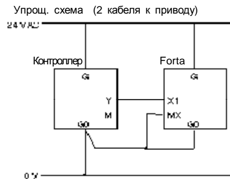
Аналог. управление, 24 V AC питание для контроллеров (TAC 239W, TAC 6711, TAC Xenta, TAC 8000, TAC 230U, TAC 2000, TAC 9000, TAC 77xx)
