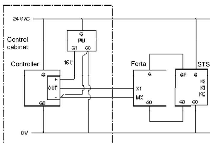
Аналоговое упр., выход контроллера с гальван. развязкой (TAC 6501, TAC 6505)
