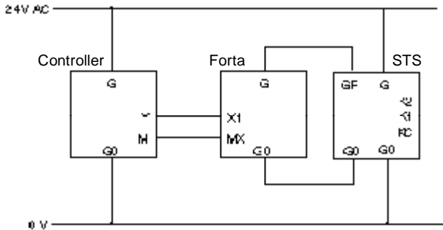
Аналог.управление, 24 V AC питание для контроллеров (TAC 239W, TAC 6711, TAC Xenta, TAC 8000, TAC 230U, TAC 2000, TAC 9000, TAC 77x)
